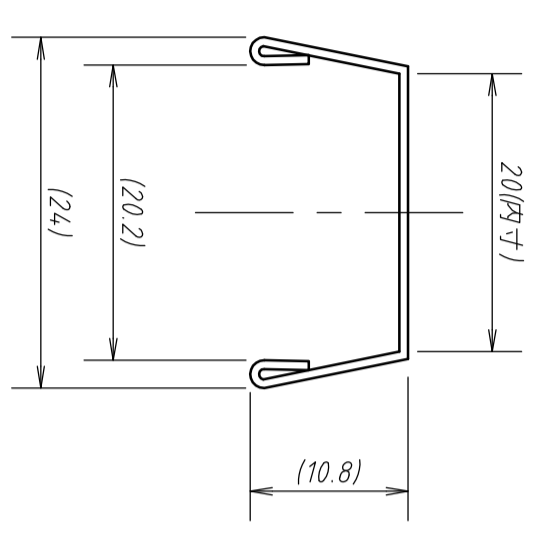
側面図 (4:1)
